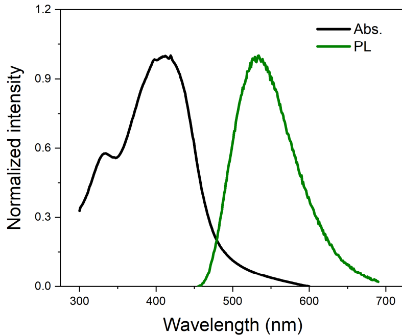
水溶剂绿光量子点吸收光谱、光致荧光曲线图
