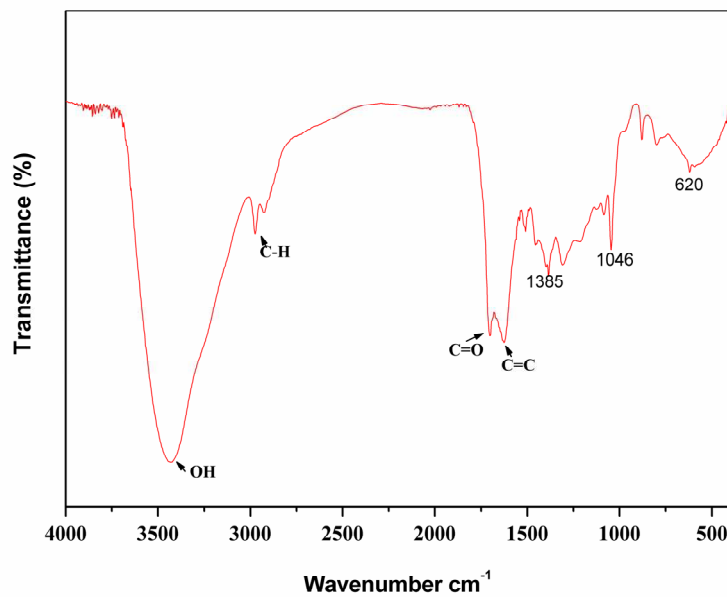
纳米空心碳球红外图
