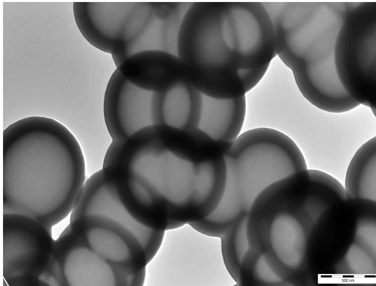
纳米空心碳球 TEM 图
