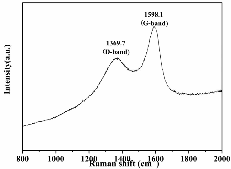
羧基化碳纳米球拉曼光谱图
